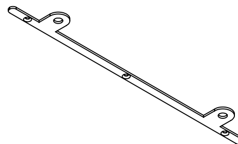
U40-04-19 Sigill fastsättningsbeslag, för soffa eller bänk Kommer monterade på möblerna ifall de önskas för fastsättning (ange /N)
